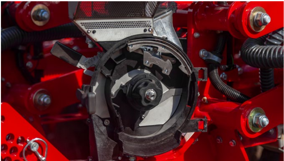
Dosador com sigulador universal
