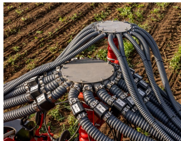
Torre de distribuição de fertilizante e microgranulados
